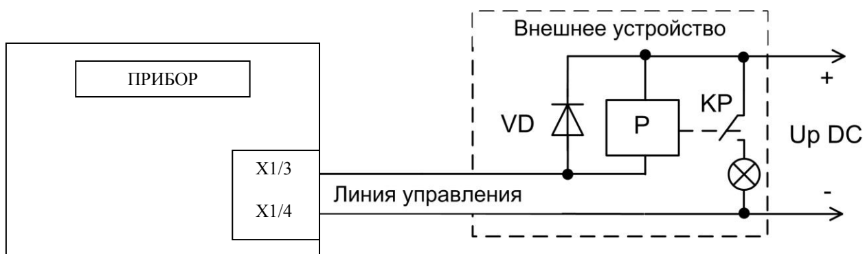
Рис.6.2. Подключение внешних устройств к прибору.
