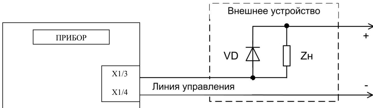
Рис.6.1. Подключение внешних устройств к прибору.
